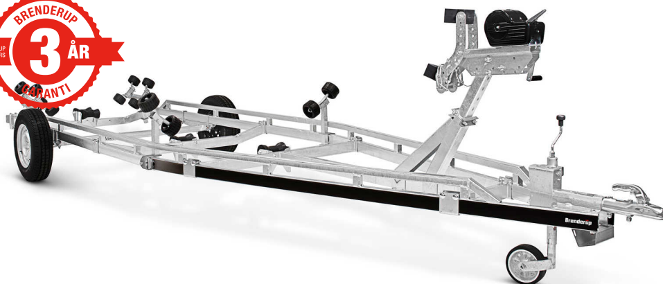
Superrullsvagga
