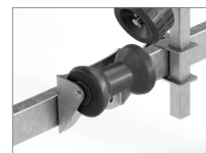
Förstärkta kölrullar
