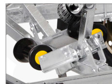
Förstärkt kölrullsvagga
